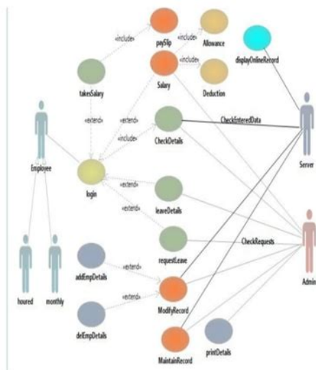
Fig: Use Case Diagram
